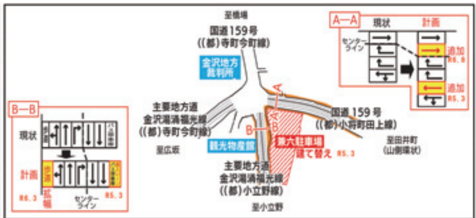
図-2 兼六園下交差点の拡幅整備
